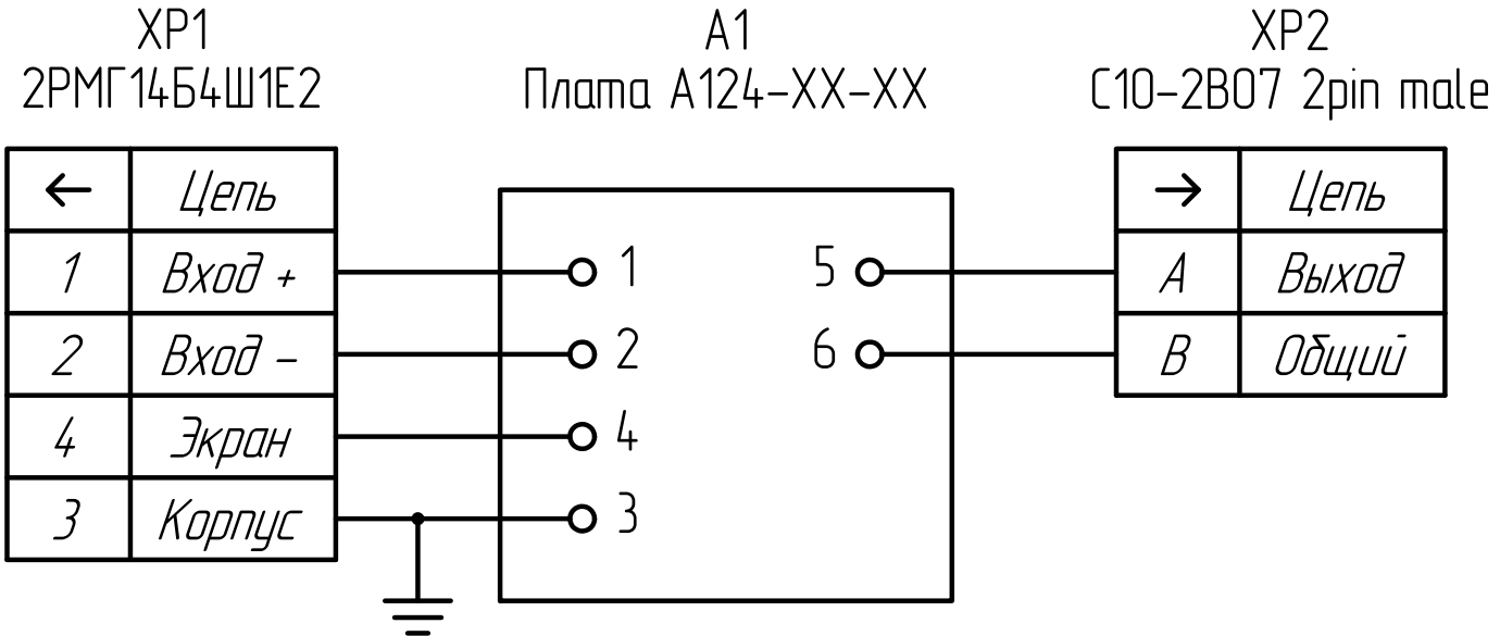
Схема электрическая соединений
