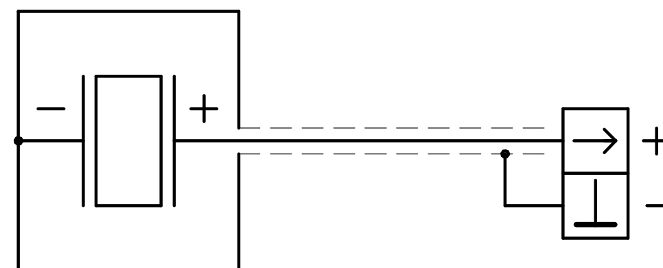
Схема электрическая
