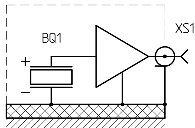
Схема электрическая принципиальная для исполнения ГТБВ.433633.018-01
