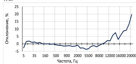
АЧХ
