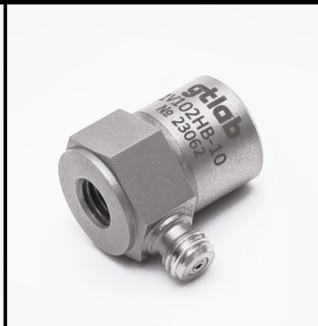
Акселерометр IEPE 1V151HC-XX
