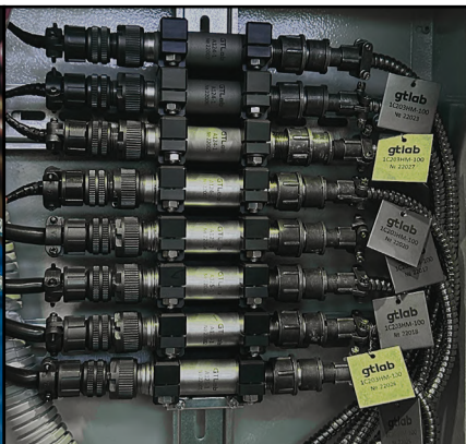
Установка формирователей А124
