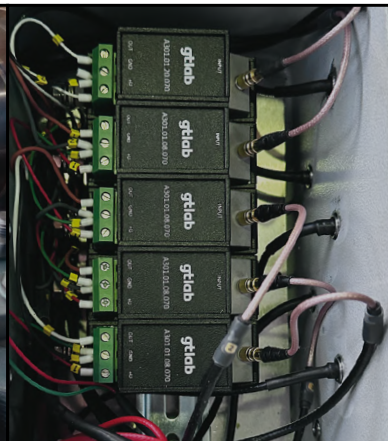
Монтаж вихрековых формирователей А301 во взрывозащищенном корпусе
