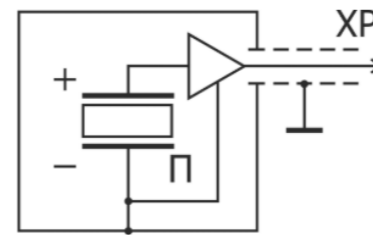
Схема электрическая соединений с доковым выходом встроенного кабеля
